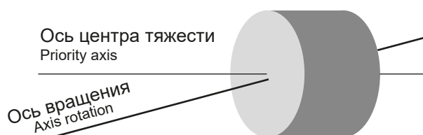
Динамическая разбалансировка Dynamic unbalance
