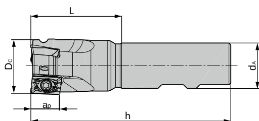
Концевая фреза 90° / AP.T 10.. End milling cutter 90° / AP.T 10..
