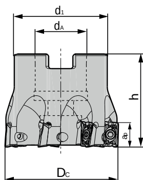
Насадная фреза 90° / AP.T 10.. Face milling cutter 90° / AP.T 10..
