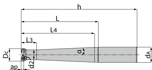
Концевая фреза конической формы A End milling cutter conical form A
