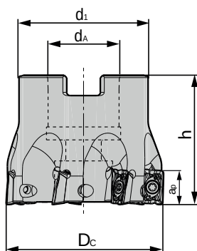
Насадная фреза 90° / AP.T 16 Face milling cutter 90°/ AP.T 16
