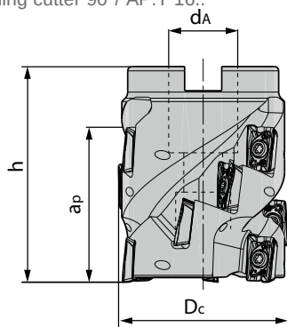
Насадная кукурузная фреза 90° / AP.T 16.. Face milling cutter 90° / AP.T 16..
