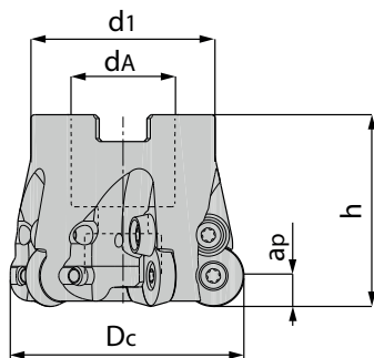
Насадная фреза Face milling cutter
