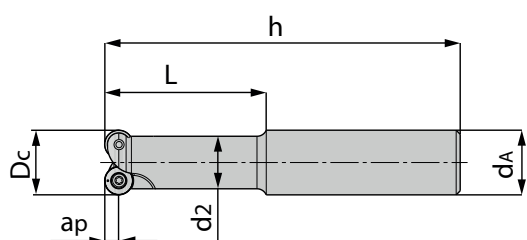
Концевая фреза цилиндрической формы B End milling cutter cylindrical form B
