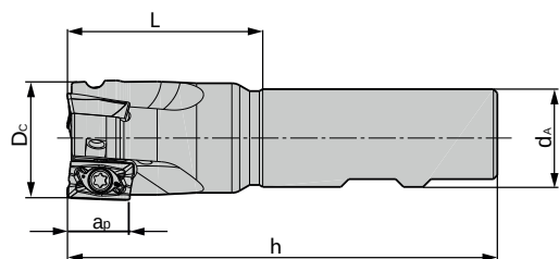
Концевая фреза 90° / AP.T 16 End milling cutter 90° / AP.T 16
