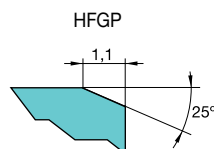
Геометрия заходной части
