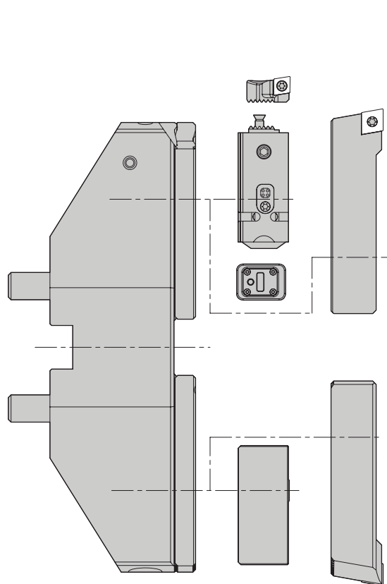
eBore — мост типоразмера S (малый)
