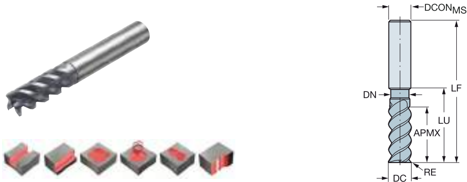
Метрическое исполнение
