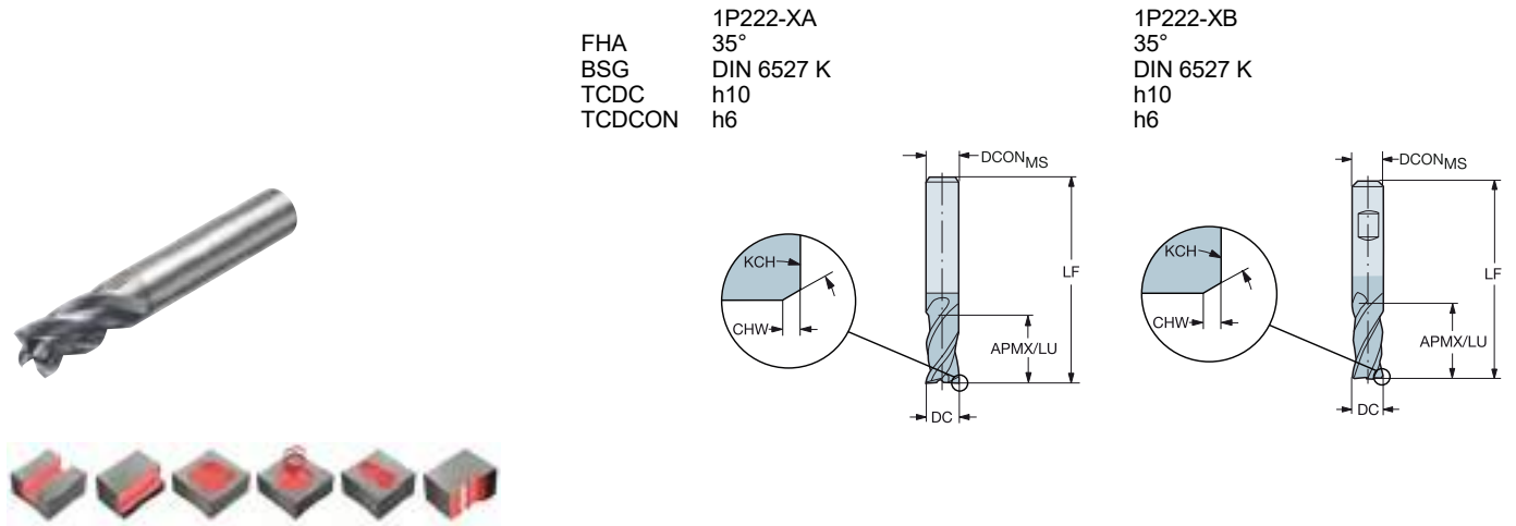
Метрическое исполнение
