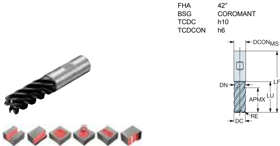
Метрическое исполнение
