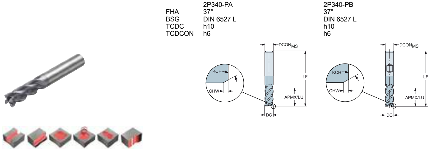
Метрическое исполнение
