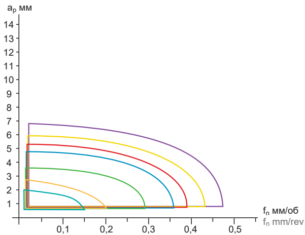
Продольное точение 12,25D Longitudinal turning 2,25D
