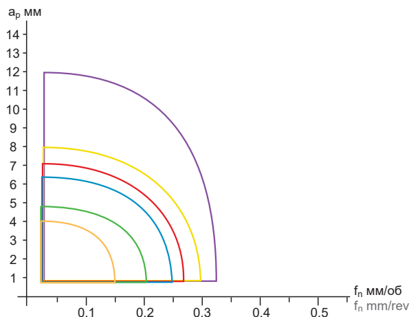
Продольное точение 1,50D Longitudinal turning 1,50D
