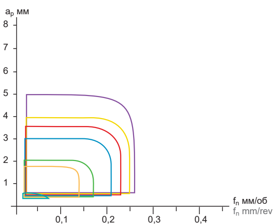
Подрезка торца 2,25D Face turning 2,25D
