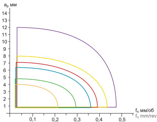
Продольное точение 11,50D Longitudinal turning 1,50D
