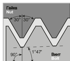
Резьба NPTF - полный профиль NPTF - Full Profile
