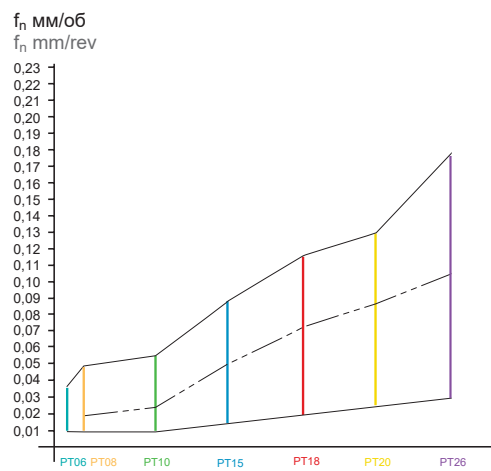
Сверление 1,50D/2,25D Drilling 1,50D/2,25D
