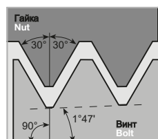
Резьба NPT - полный профиль NPT - Full Profile
