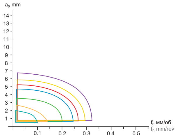
Продольное точение 2,25D Longitudinal turning 2,25D
