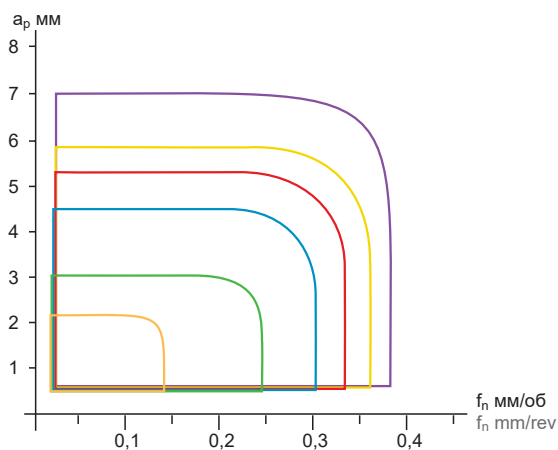
Подрезка торца 1,50D Face turning 1,50D
