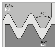
Неполный профиль 60° Partial Profile 60°
