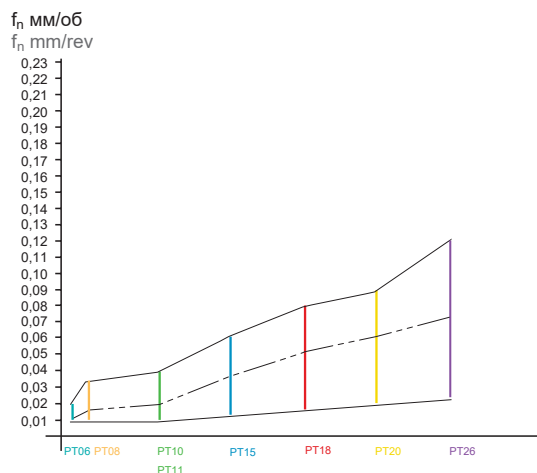
Сверление 1,50D/2,25D Drilling 1,50D/2,25D
